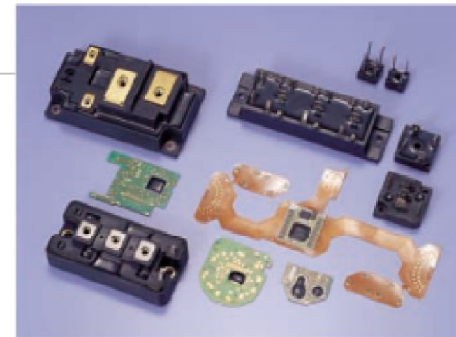
液状エポキシ樹脂製品が使用されている個別半導体製品、COB Various discrete semiconductors and COB, insulated by liquid epoxy product.
